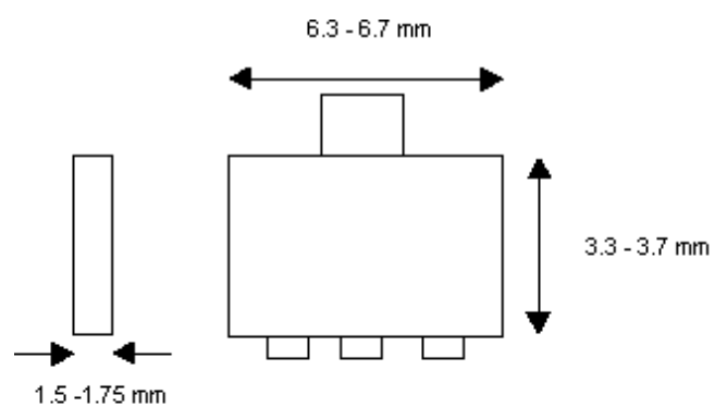
SOT- 223
